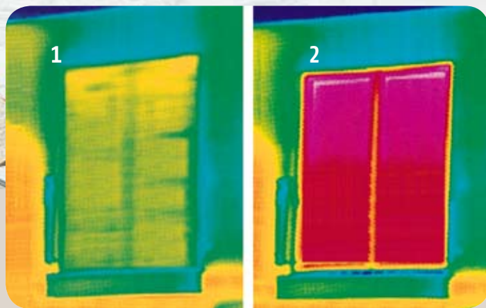
Bei einem Fenster mit geschlossenen Rollläden (1) ist die Wärmedurchlässigkeit deutlich geringer gegenüber einem Fenster mit hochgezogenen Rollläden (2).
