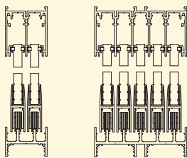
Vertikalschnitt: 2-gleisige Anlage und 5-gleisige Anlage
